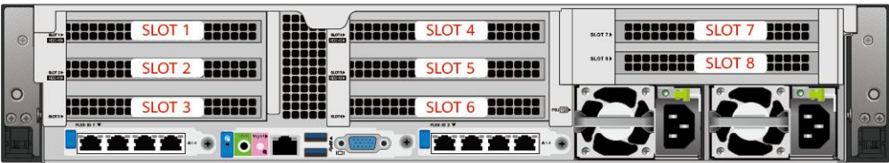
图 5-15 8 个 PCIe 插槽
