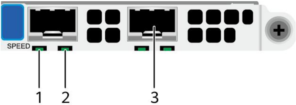
图 5-17 SF223D-H（2x25GE 光口）
