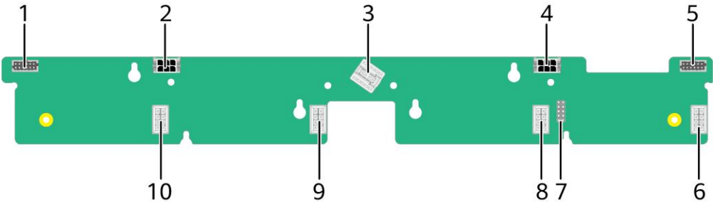
图 5-6 风扇板接口
