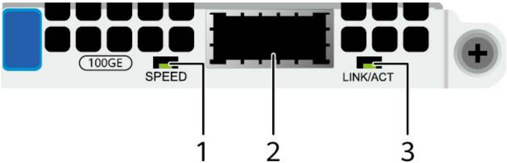
图 5-18 SF225S-H（1x100GE 光口）
