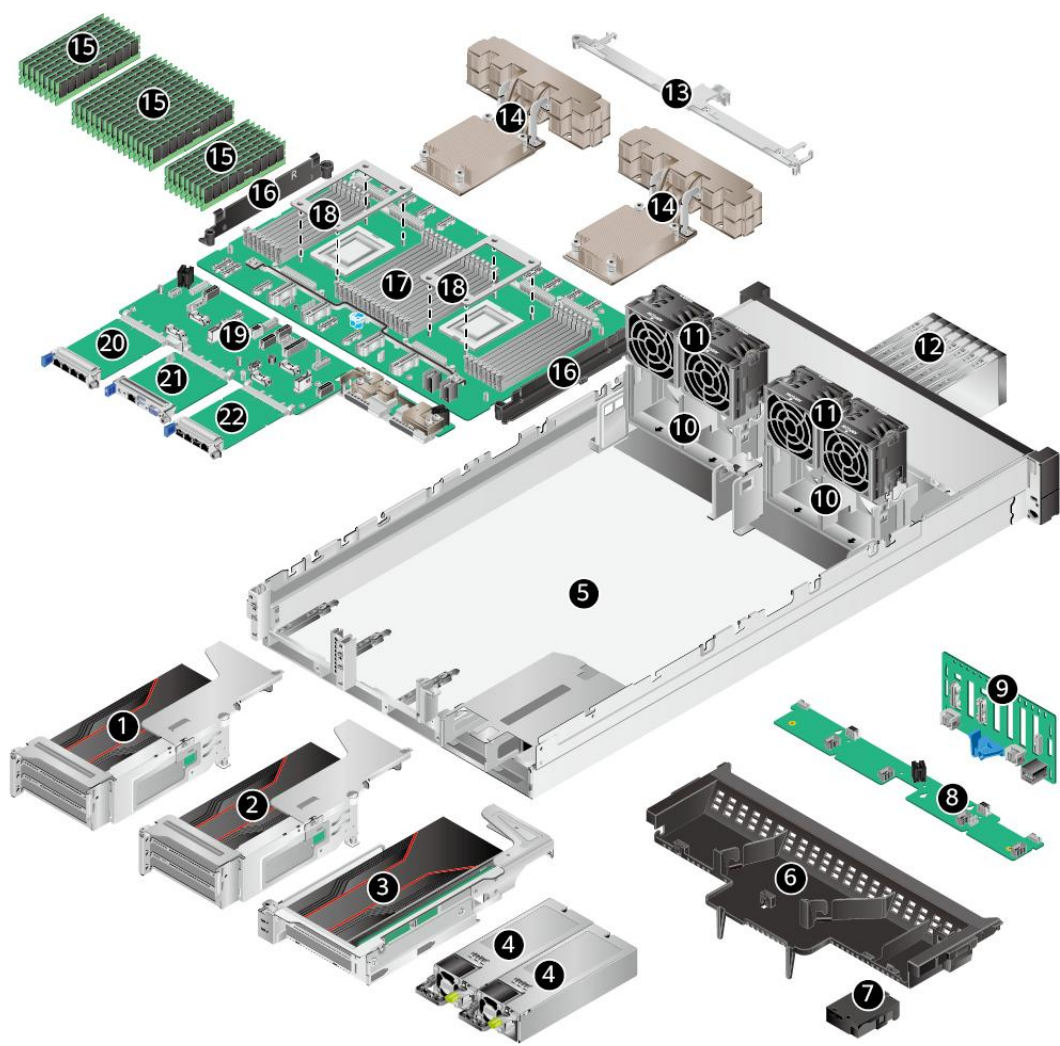
图 3-1 部件
