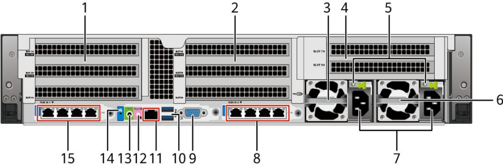
图 5-2 后面板
