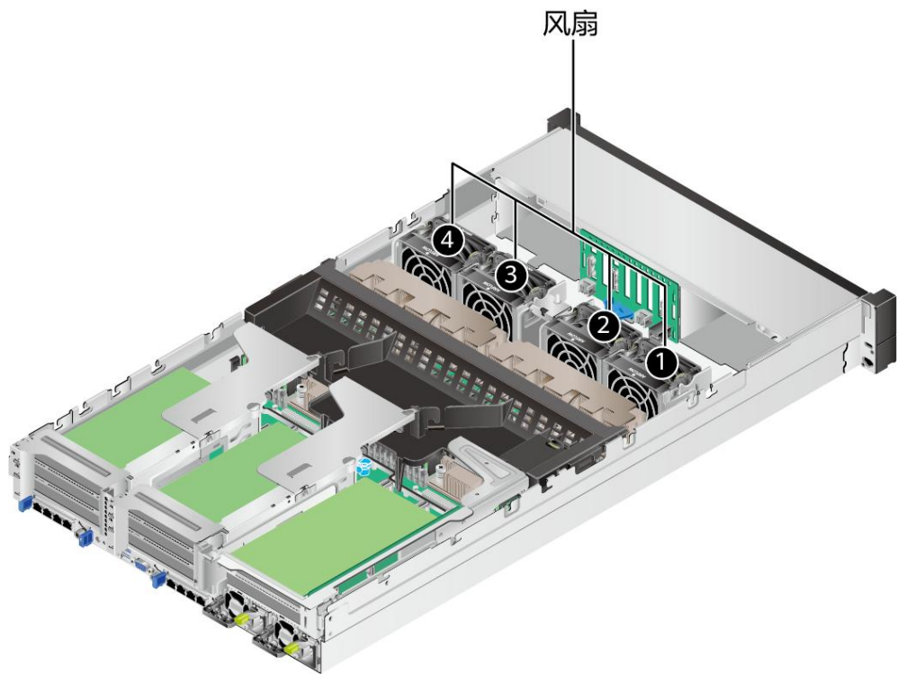
图 5-7 风扇位置图
